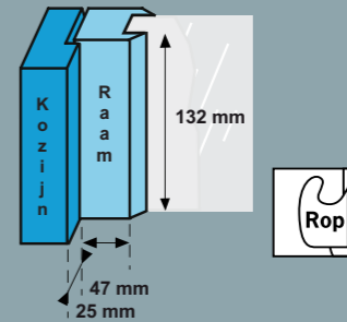
Benodigde montage ruimte Met opbouwsluitkom Met onderlegplaat Naar buitendraaiend
